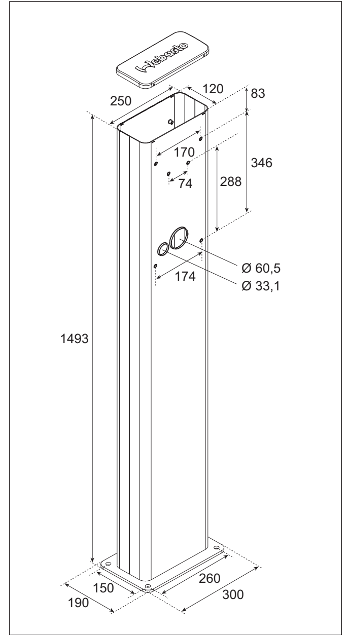
Fig. 04: Stand dimensions
